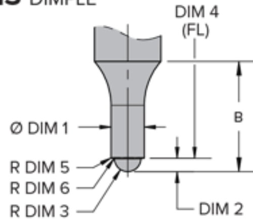
R13 DIMPLE
